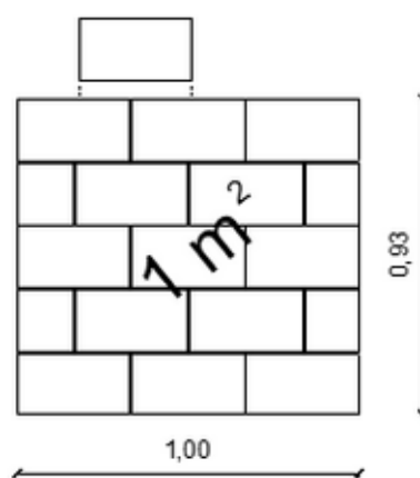
Con adhesivo - 16 ladrillos
