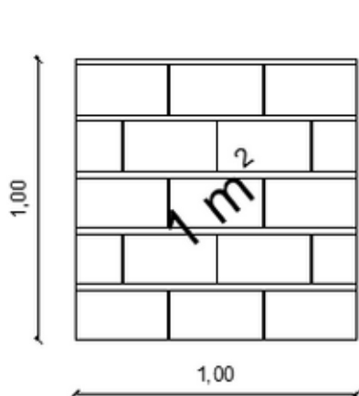
Con mortero - 15 ladrillos
